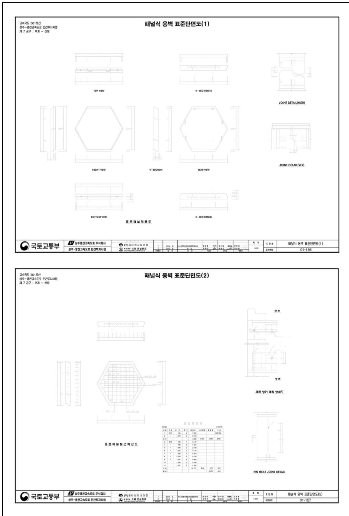
【그림 11.6】 단면도(계속)
